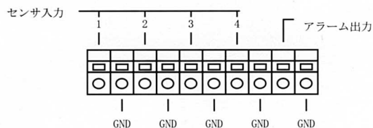
端子台ピン配置図
