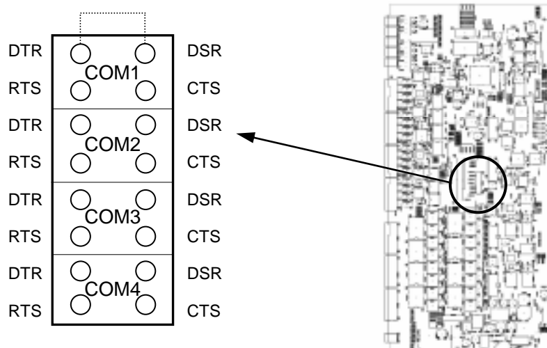
本体の B20265 基板中央のジャンパーコネクタ( S6001 )
